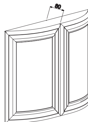
Пара закругленных дверок 716 X 446,5
